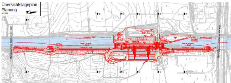
Übersichtslageplan neue Schleuse
